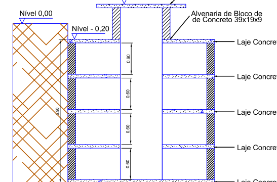
CORTE CC Sem Escala
