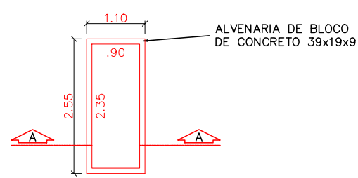
PLANTA BAIXA CARNEIRAS esc 1:100
