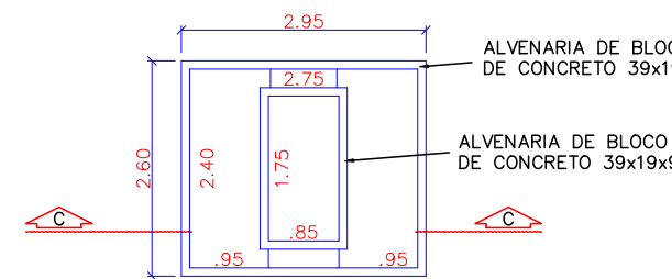
PLANTA BAIXA JAZIGO 8 LUGARES esc 1:100
