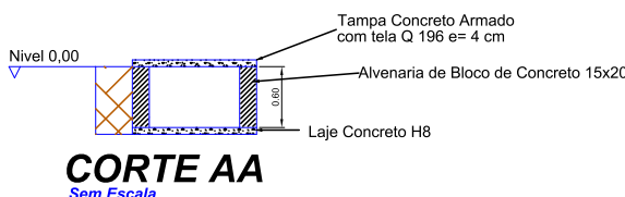
CORTE AA Sem Escala
