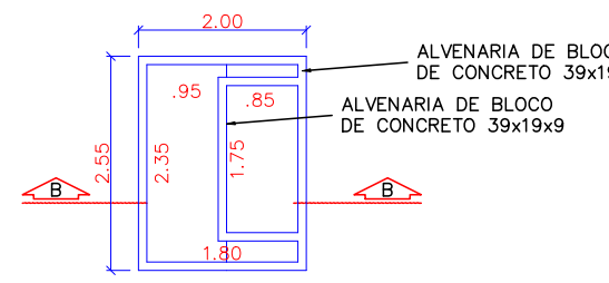
PLANTA BAIXA JAZIGO 3 LUGARES esc 1:100
