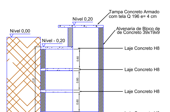
CORTE BB Sem Escala
