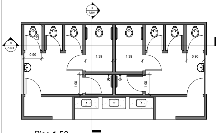
1 Piso 1 50 1 : 50
