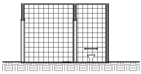
3 Corte 2 1 : 50
