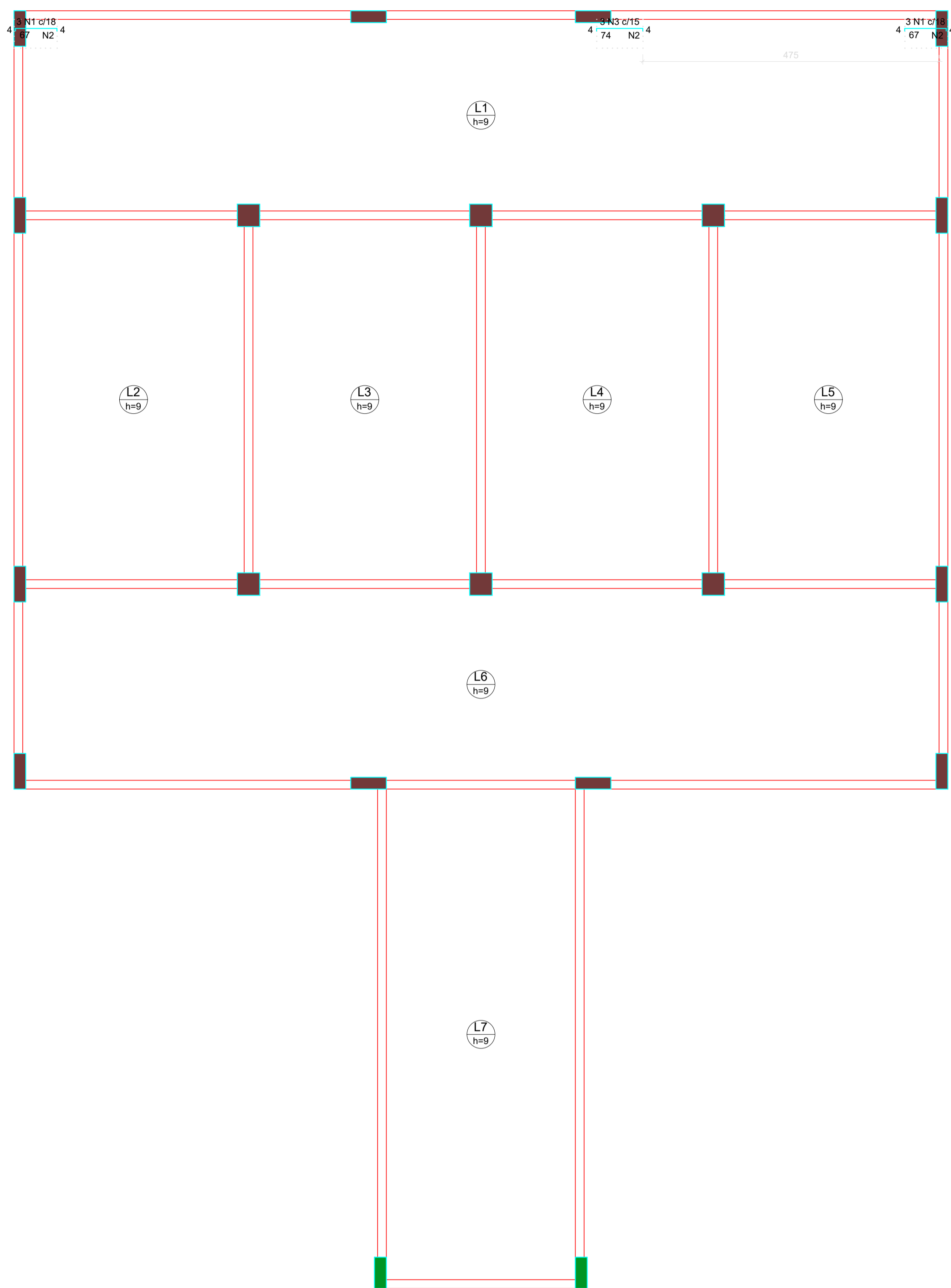
Armação negativa das lajes do pavimento Terreo (Eixo X) escala 1:50
