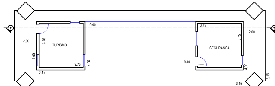
PLANTA BAIXA ATUAL Esc.: 1/100
