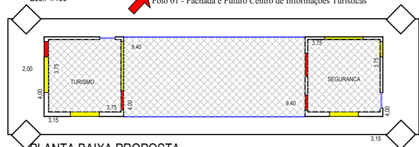
PLANTA BAIXA PROPOSTA Esc.: 1/100
