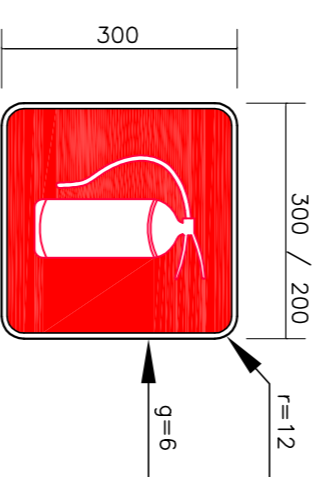
02 PLACAS DE SINALIZAÇÃO DE EXTINTOR SEMI ESCALA
