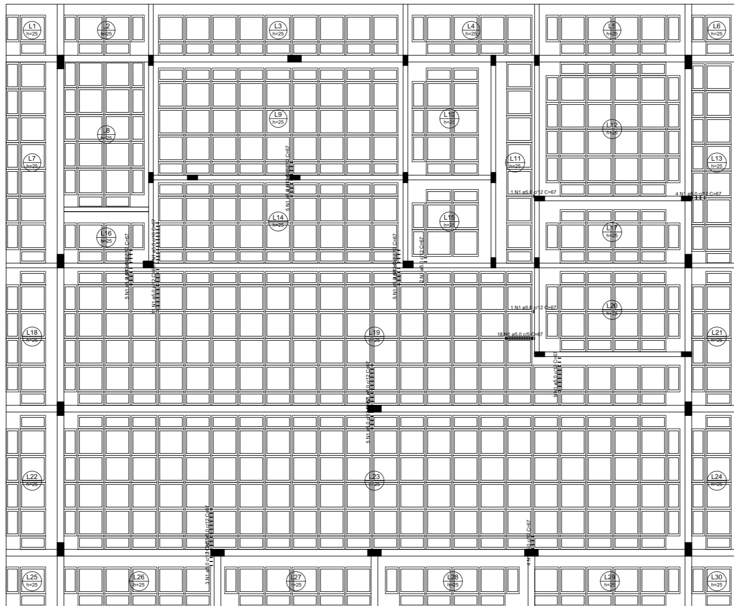
Detalhamento de punção e cisalhamento das lajes do pavimento COBERTURA (Nível 400) escala 1:50
