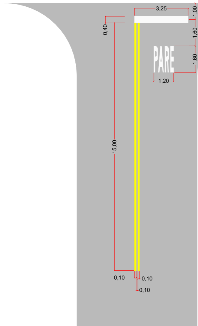
Detalhamento Sinalização Horizontal Escala 1:200
