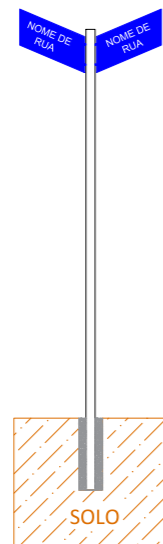
PLACA DE IDENT. DE RUA Vista Lateral Escala 1:50
