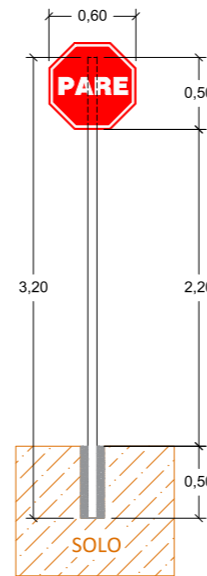
PLACA R1 Vista Frontal Escala 1:50
