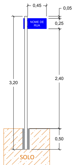
PLACA DE IDENT. DE RUA Vista Frontal Escala 1:50
