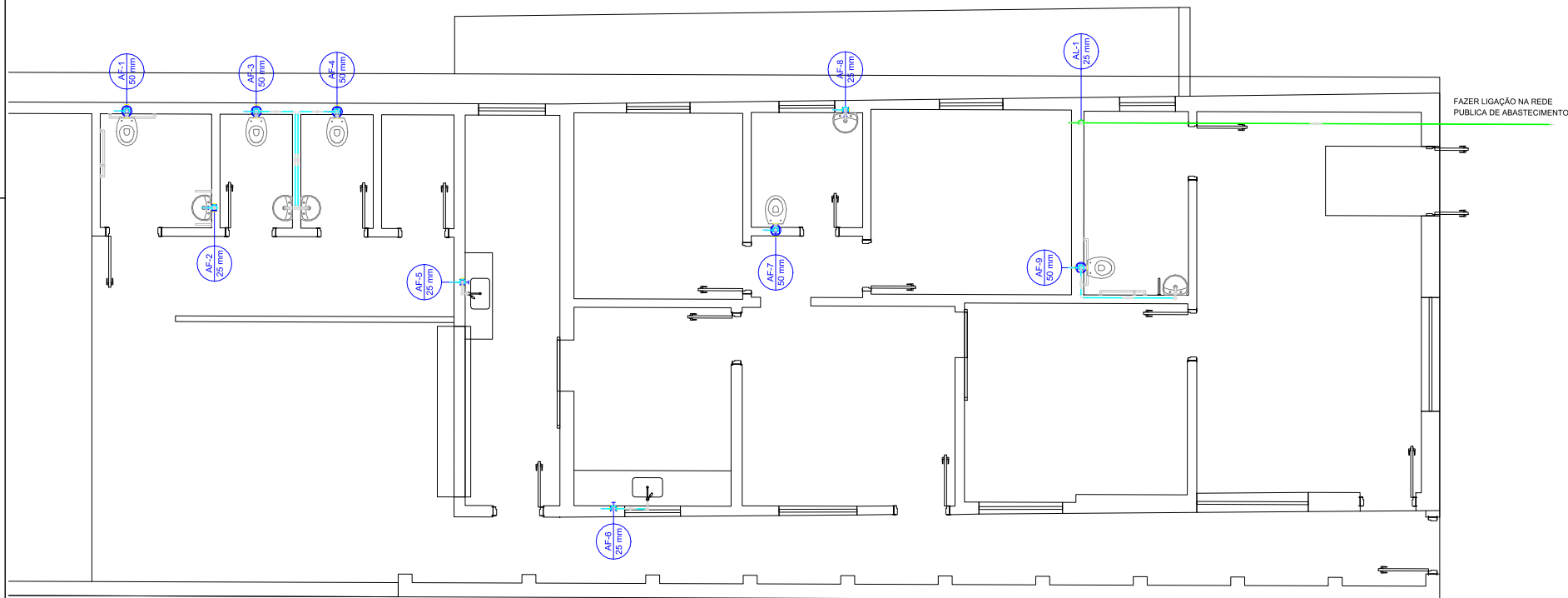
Planta Baixa - Água Fria Escala 1:50
