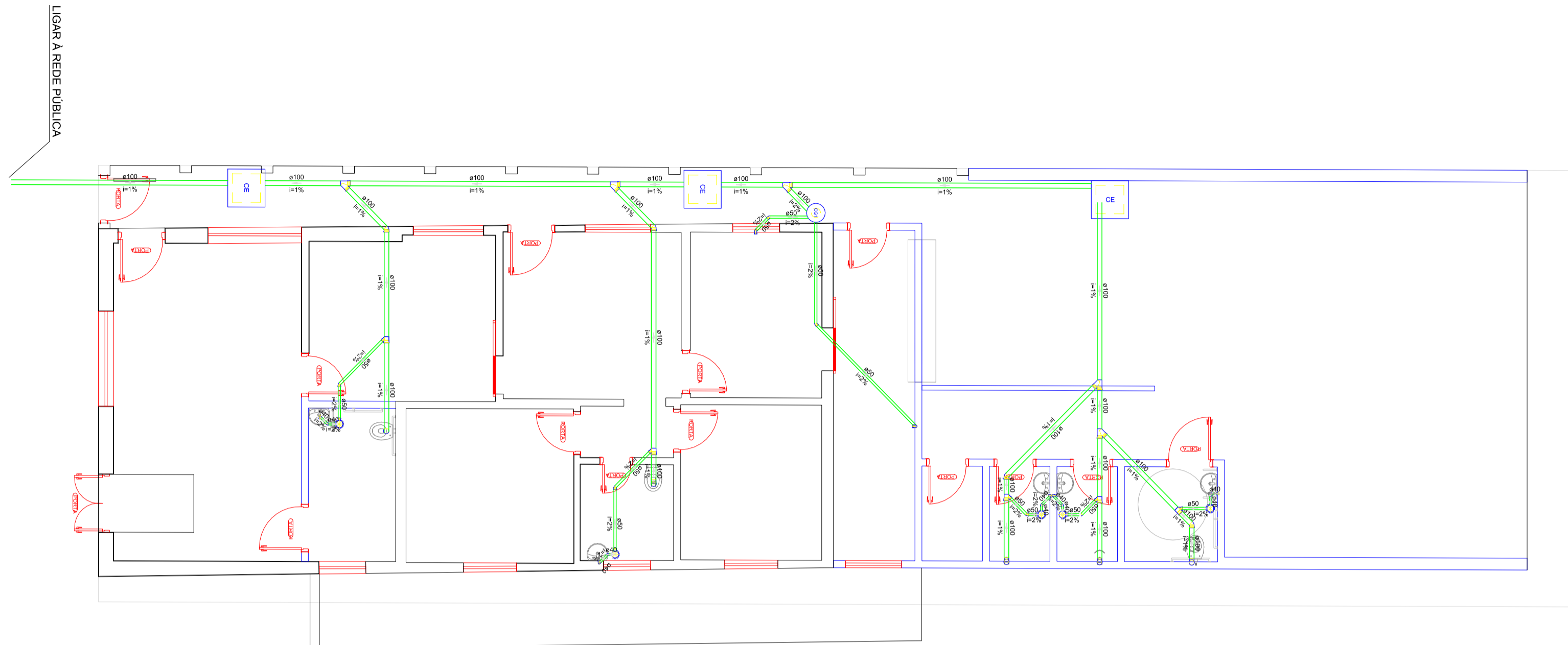
INSTALAÇÕES HIDROSSANITÁRIA ESGOTO ESCALA: 1:755
