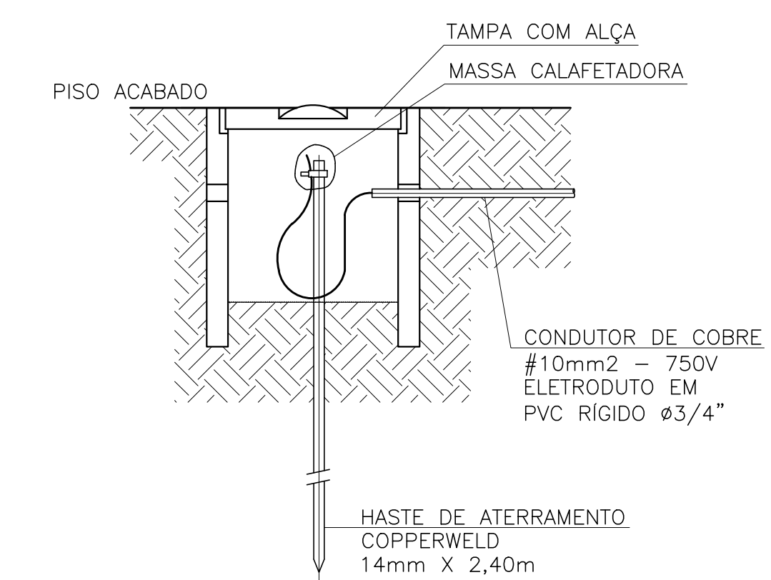
CAIXA DE INSPEÇÃO DE ATERRAMENTO SEM ESCALA
