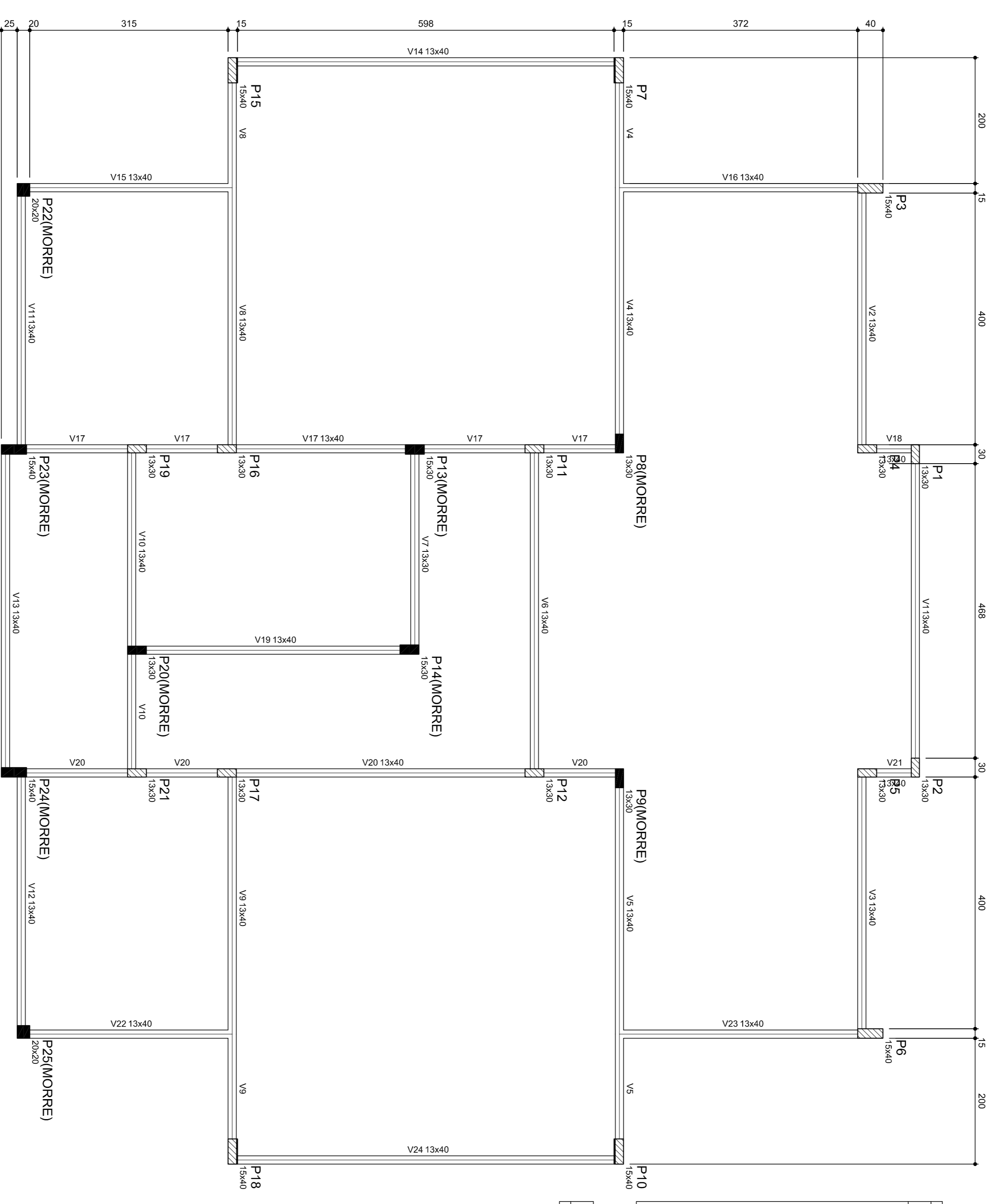
Forma do pavimento Nivel 000 escala 1:50
