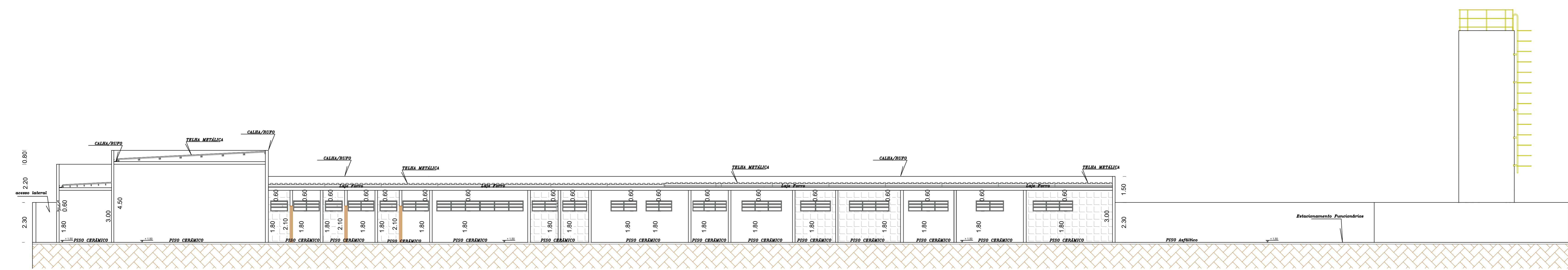
Corte BB Escala: 1:100
