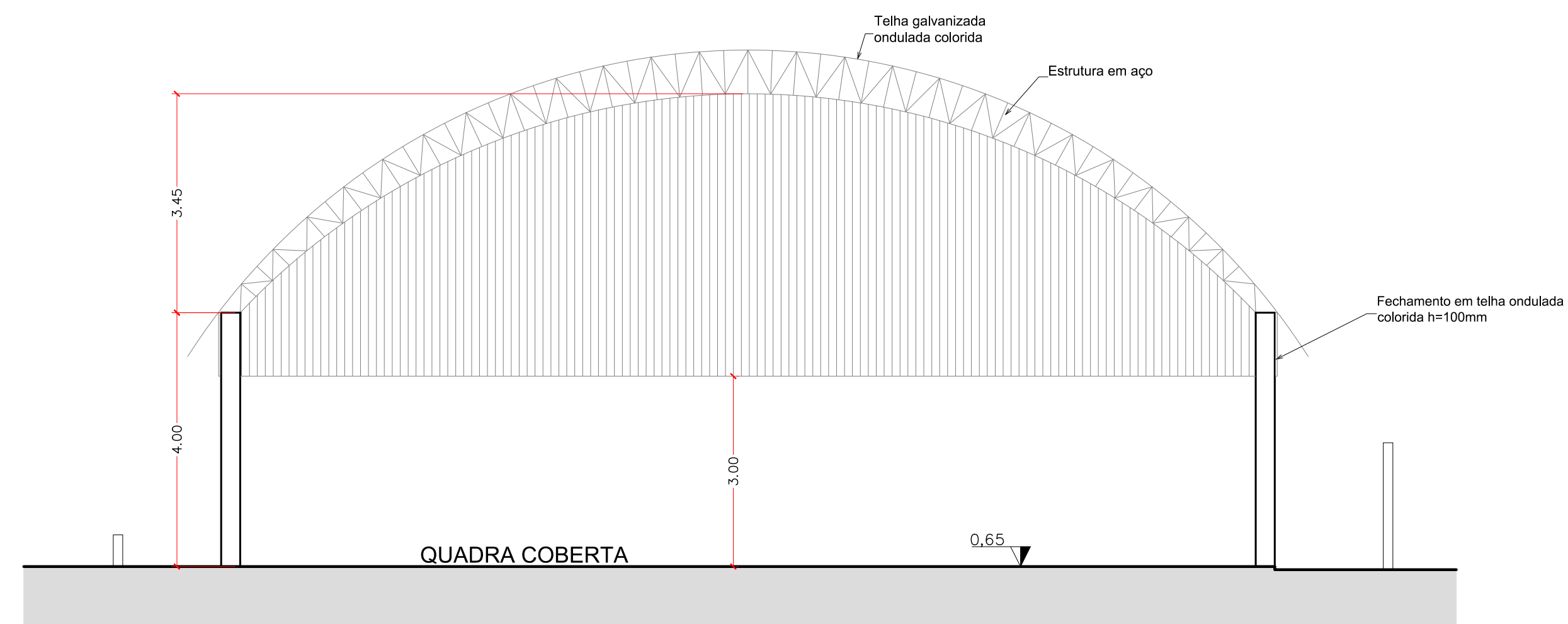
CORTE CC BLOCO D - QUADRA COBERTA ESCALA 1:75
