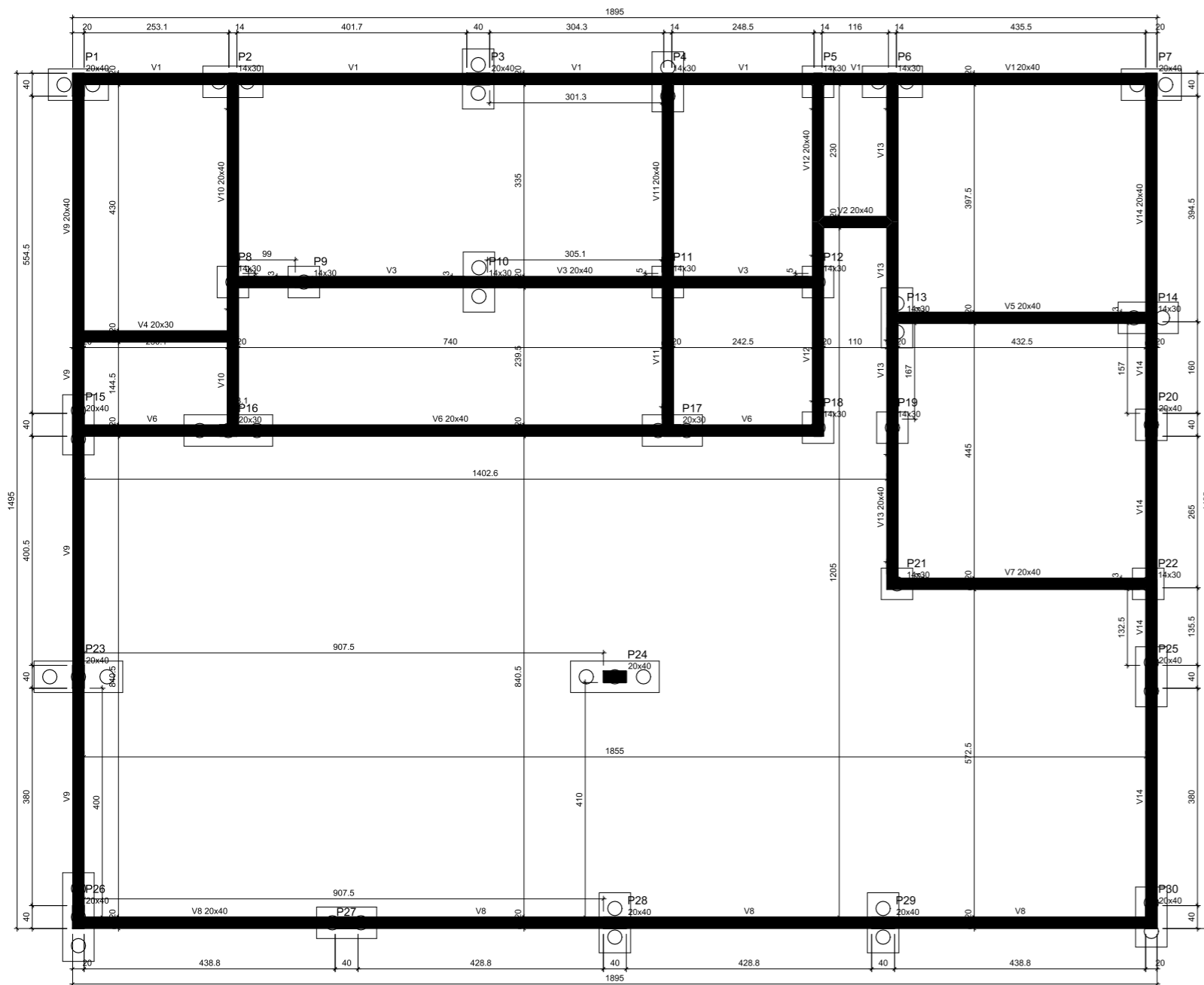
Forma do pavimento FUNDAÇÃO (Nível 0) escala 1:50
