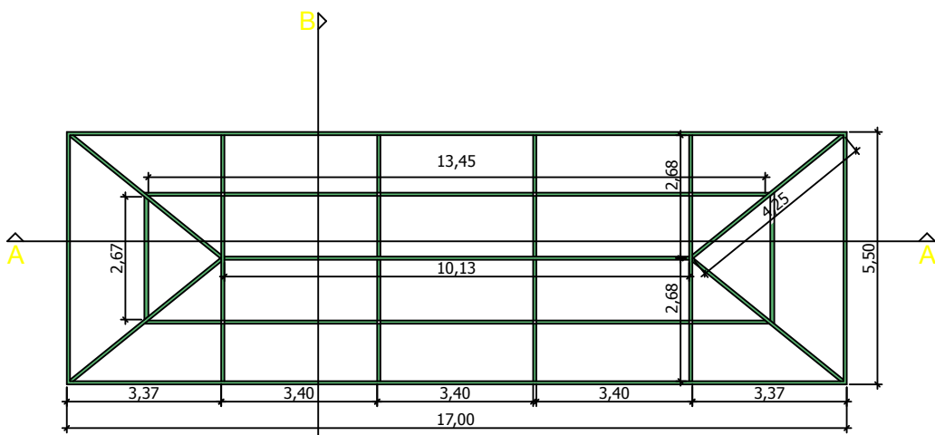
PLANTA BAIXA
